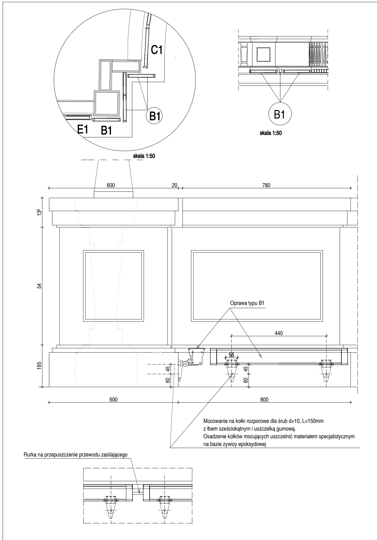
RYS 3. DETAL MOCOWANIA OPRAW TYPU "B1", "C1", "E1" DO BALUSTRAD WIADUKTU NAD PRZYCZÓŁKIEM ZACHODNIM MOSTU - SKALA 1:10
